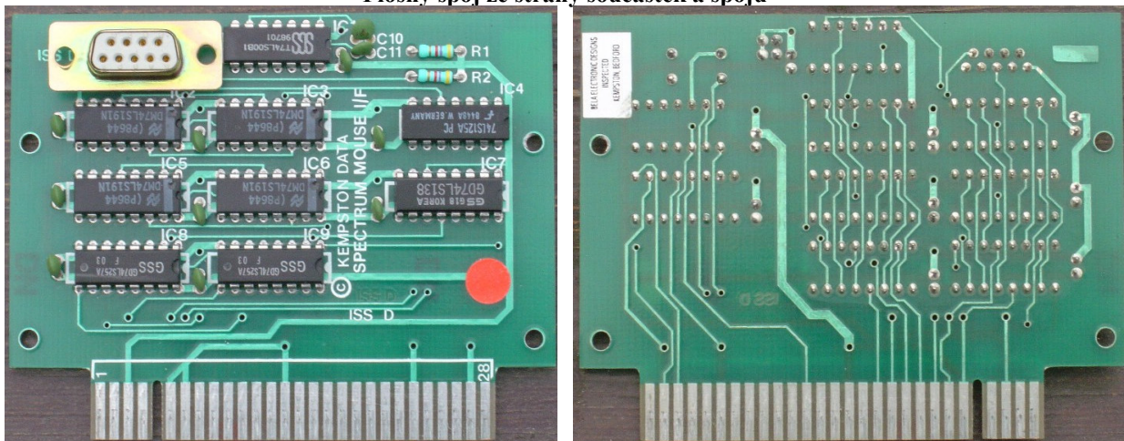
Plošný spoj ze strany součástek a spojů
